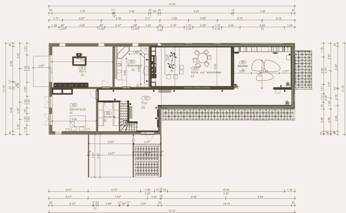
Grundriss Erdgeschoss
