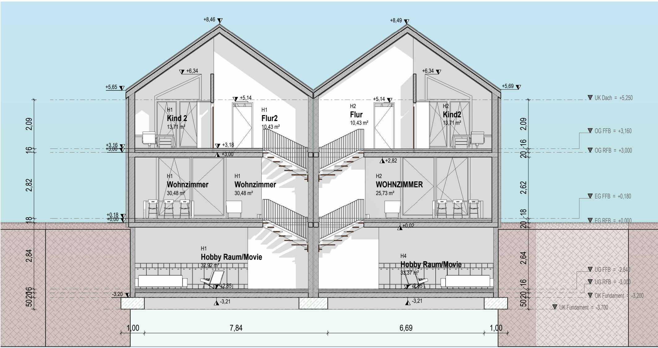
B1-2 1 : 100
