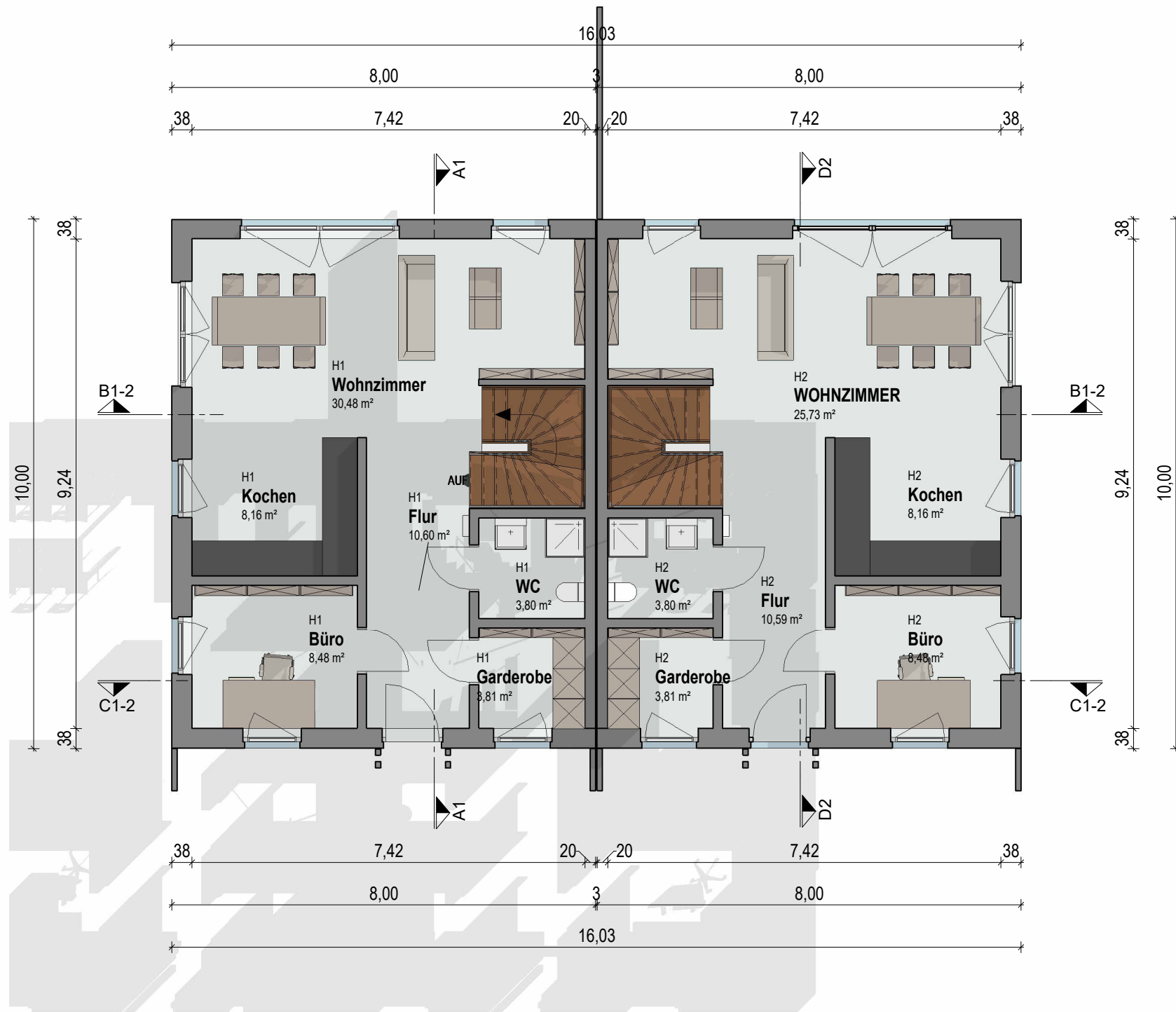
EG FFB 1 : 100
