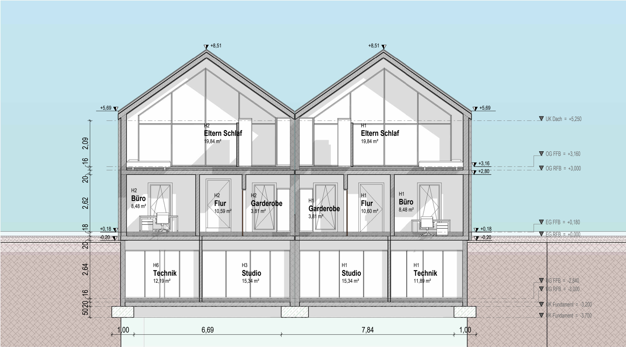
C1-2 1 : 100
