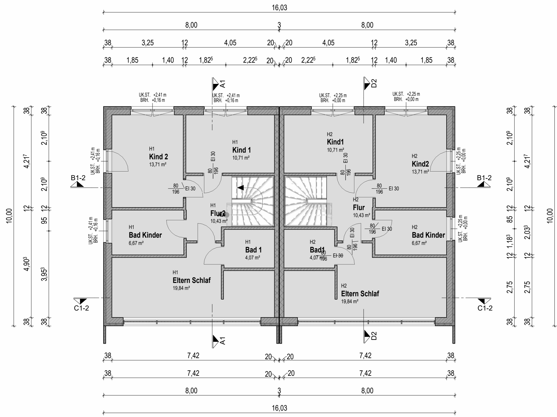
1. Obergeschoss 1 : 100
