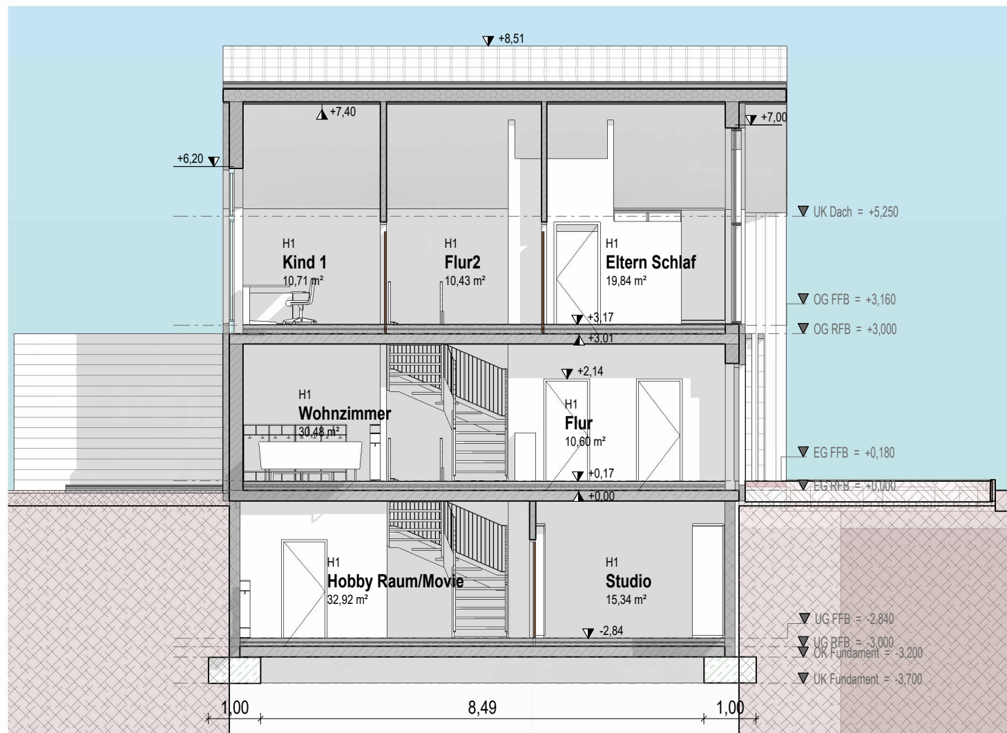
A1 1 : 100
