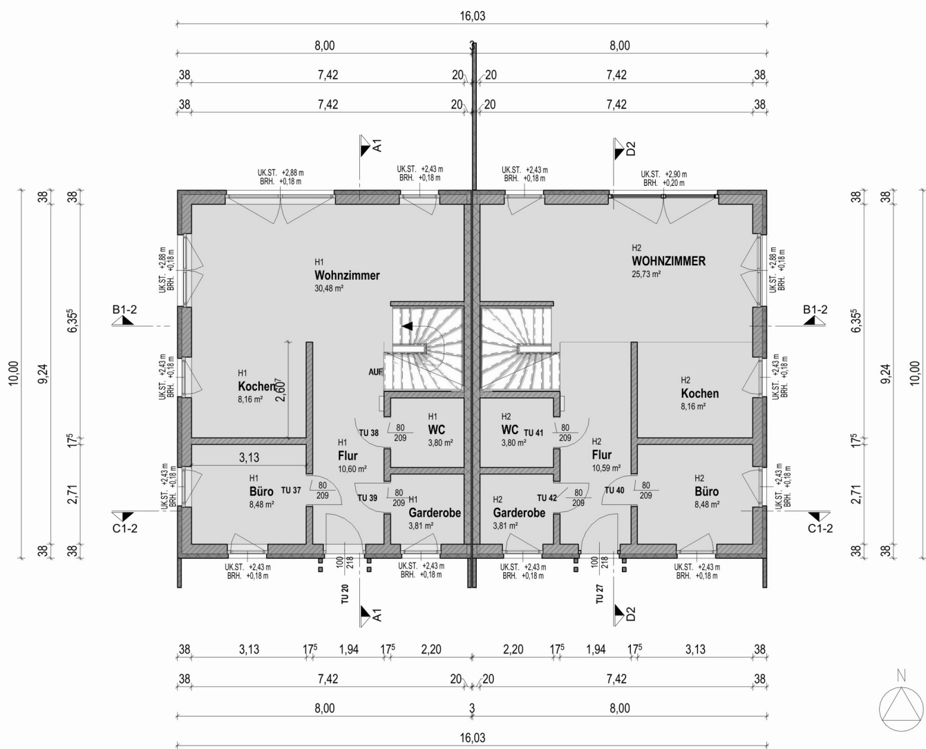
Erdgeschoss 1 : 100
