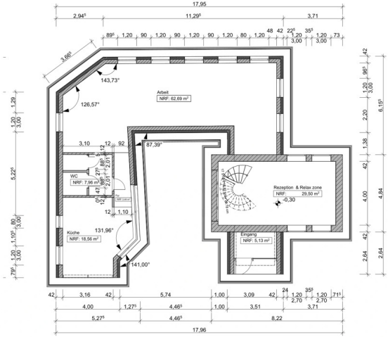
EG Endzustand / M: 1:100
