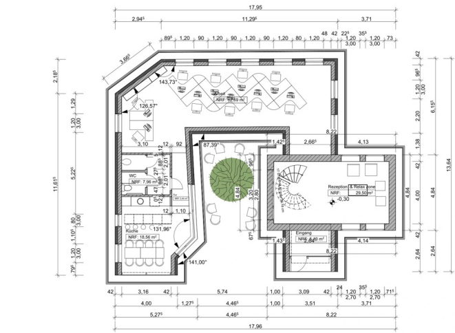
EG Möbel / M: 1:100
