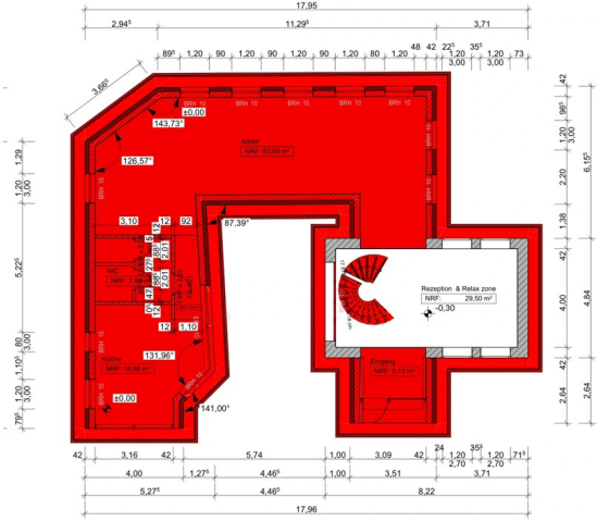
EG Endzustand / M: 1:100
